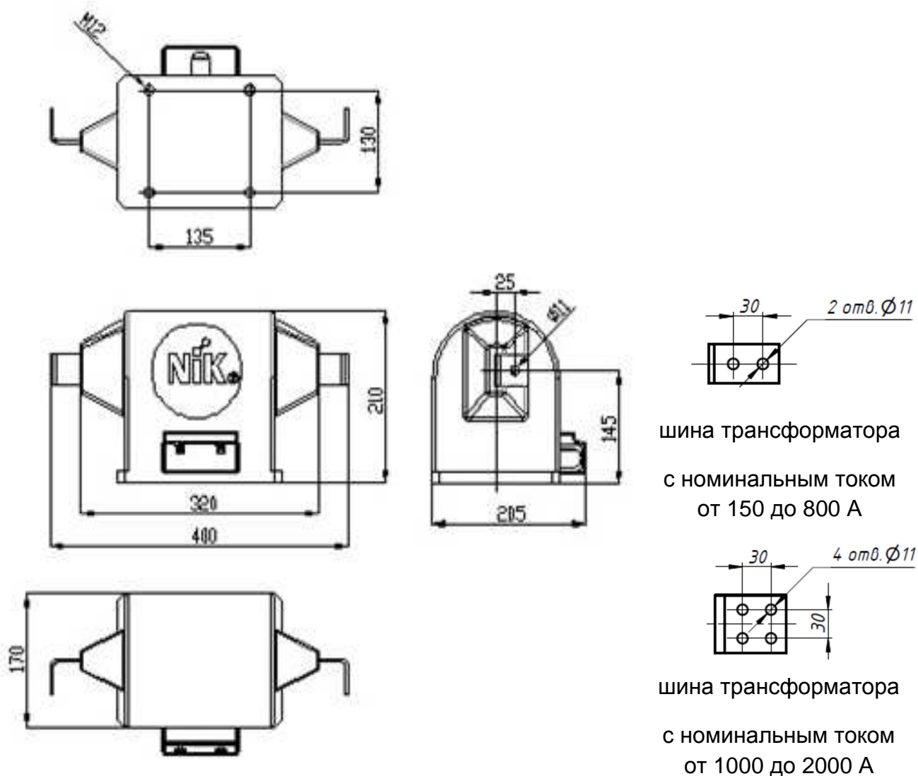
Рисунок А.1 Габаритный чертеж трансформаторов ТПЛН-10...
