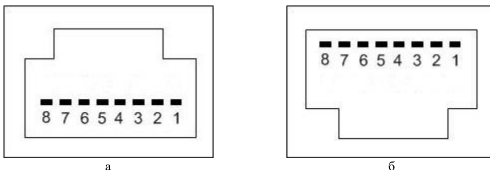
Рисунок 3 – Нумерація контактів роз'ємів M1 і M2 (типу RJ-45) першого або другого додаткових інтерфейсів
