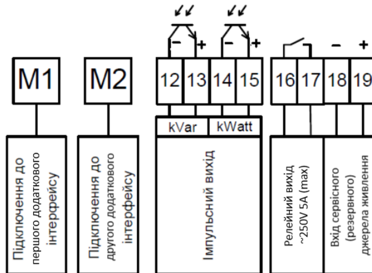
Рисунок 2 – Схема підключення інтерфейсів лічильників
