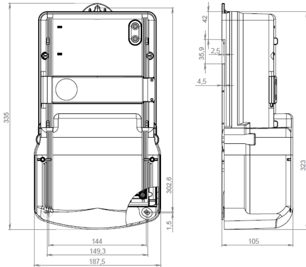
Рисунок 6. Габаритні і установочні розміри лічильника з реле відключення споживача ( див. таблицю 2.2)
