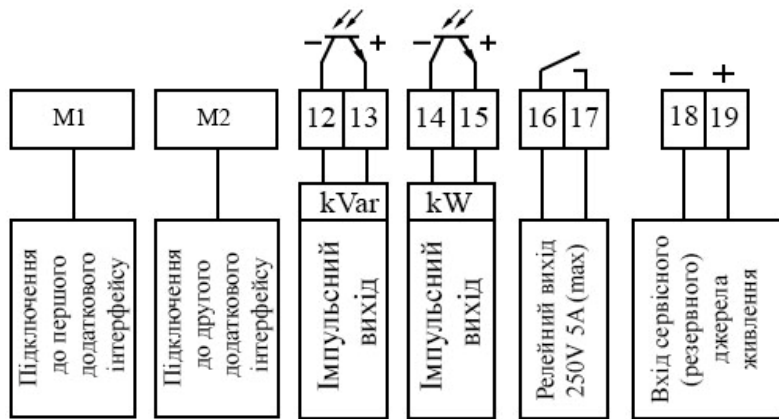
Рисунок 2 – Схема підключення інтерфейсів лічильника
