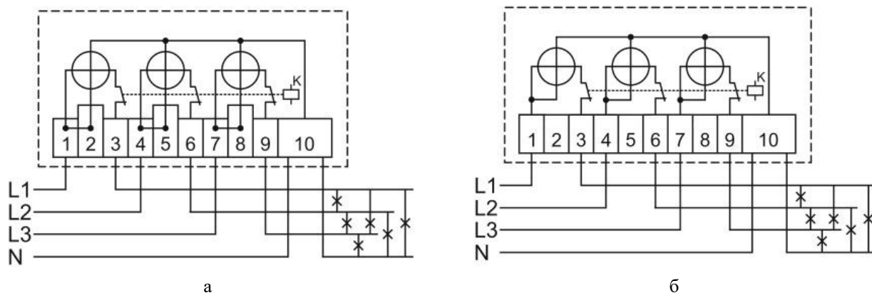
Рисунок 1 - Схема Підключення лічильників типів NIK 2307 (0.5s)...P3...
