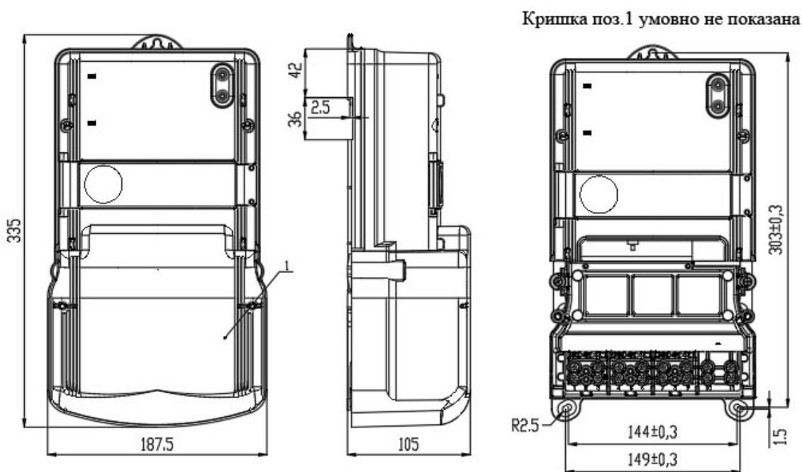
Рисунок 5 Габаритні та установочні розміри лічильника НІК2307...РЗ... з встановленим реле відключення споживача 120А
