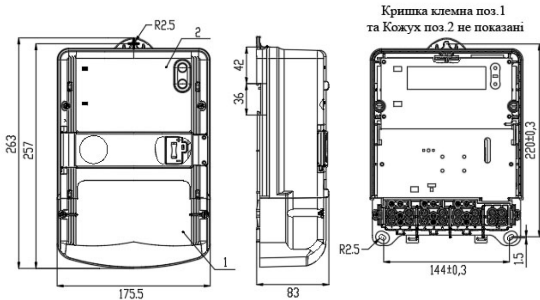
Рисунок 4 Габаритні та установочні розміри лічильника НІК2307...РЗ... без реле відключення споживача 120А
