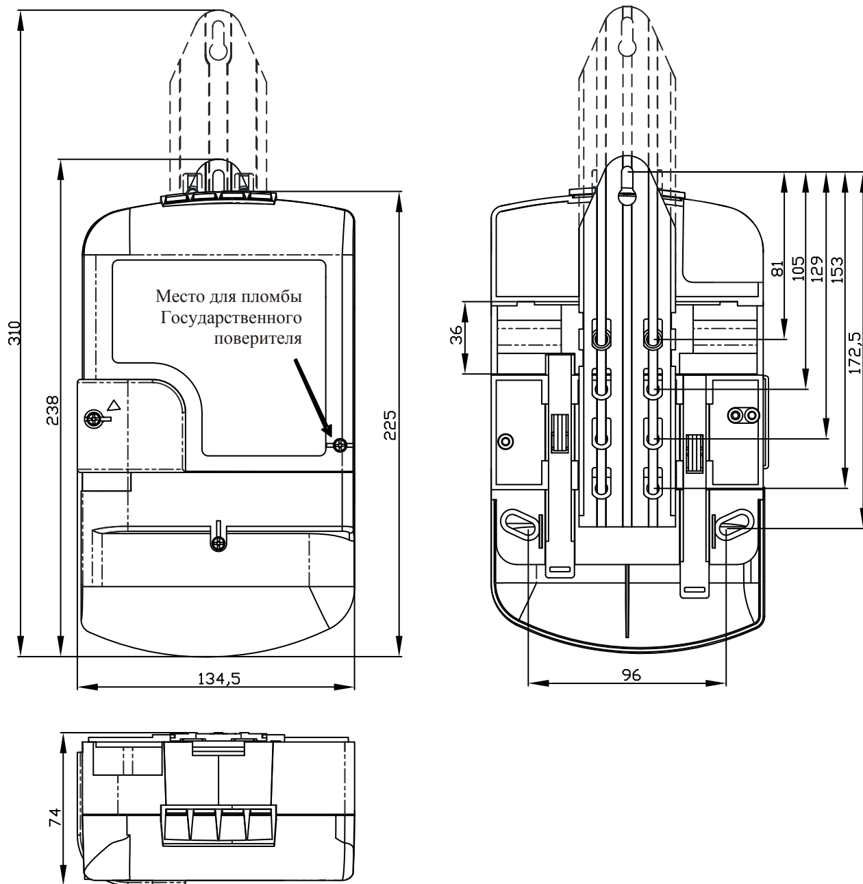
Рисунок А.1 – Габаритные и установочные размеры счетчиков НІК 2104(Р)-XX.XX.
